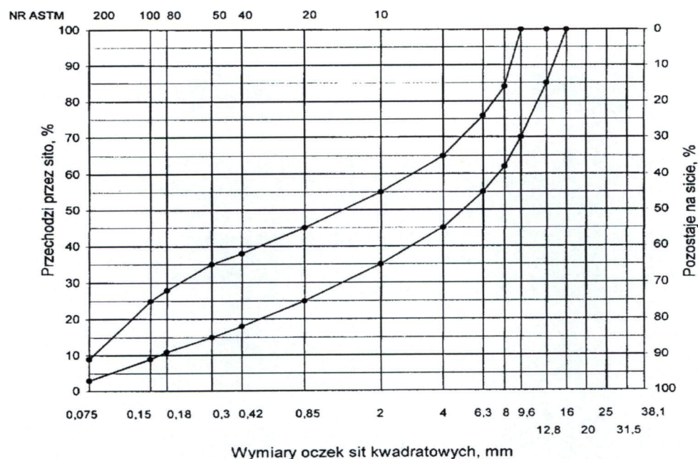
Rys. 10. Krzywe graniczne uziarnienia mieszanki mineralnej BA od 0 do 12,8 mm do warstwy wiążącej, wyrównawczej i wzmacniającej nawierzchni drogi o obciążeniu ruchem KR1 lub KR
